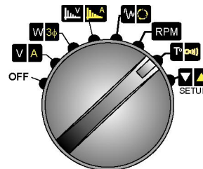
Figure 43 : Le commutateur rotatif en position T° .
