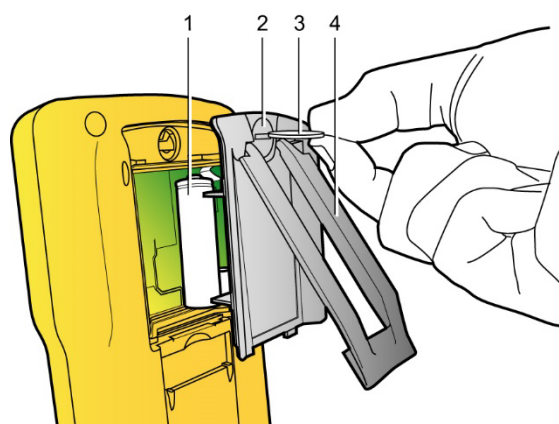
Figure 4 : Accès aux éléments de la batterie.
