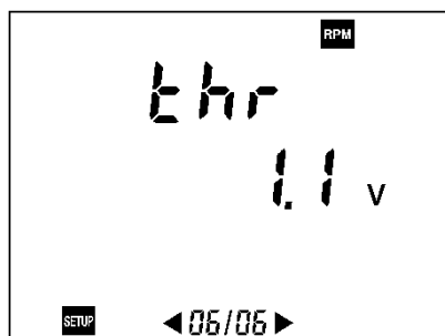
Figure 54 : Affichage du paramètre relatif à la tension de seuil du capteur tachymétrique.
