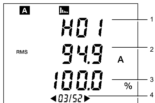
Figure 30 : Exemple d'affichage de la page 3/52.
