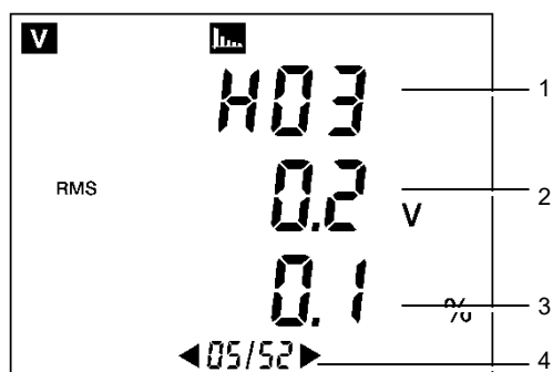
Figure 27 : Exemple d'affichage de la page 5/52.
