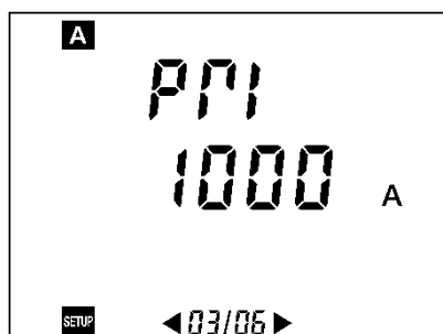
Figure 49 : Affichage du paramètre relatif au courant efficace primaire du transformateur d'intensité.
