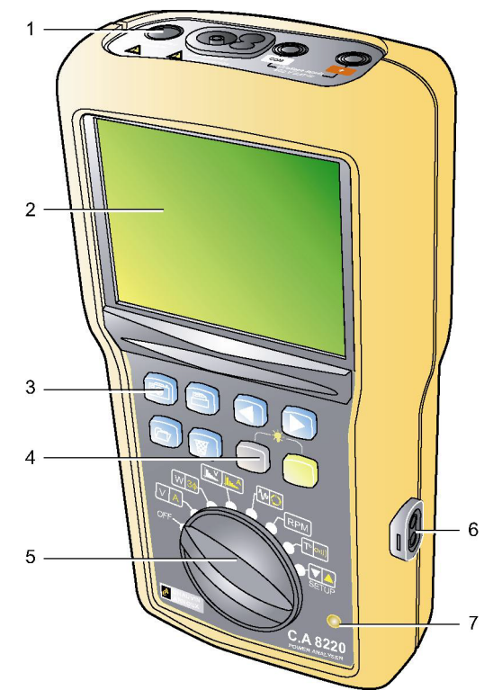
Figure 1 : Vue générale du C.A 8220.
