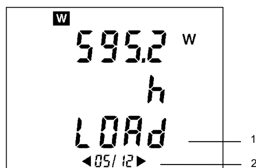
Figure 22 : Exemple d'affichage de la page 5/12.
