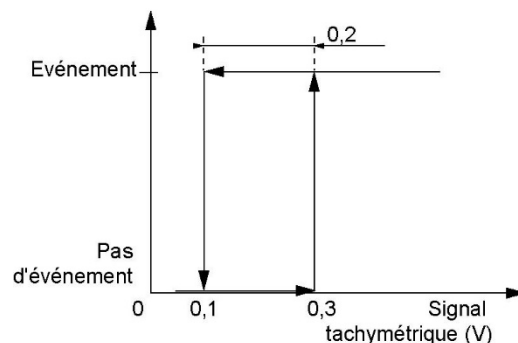
Figure 55 : Fonctions de détermination d'événement.
