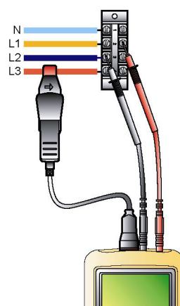
Figure 75 : Connexion en triphasé équilibré. 006
