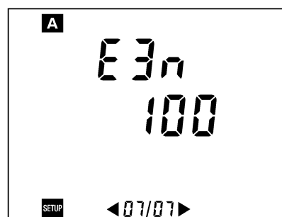
Figure 52 : Affichage du paramètre relatif à la sensibilité utilisée sur la pince.
