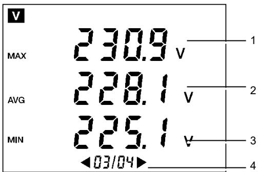
Figure 11 : Exemple d'affichage de la page 3/4.
