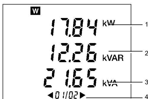
Figure 18 : Exemple d'affichage de la page 1/12.
