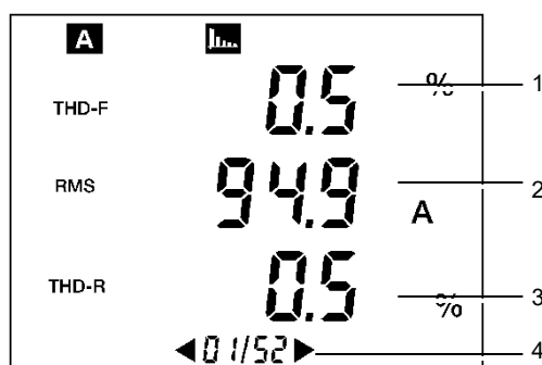
Figure 28 : Exemple d'affichage de la page 1/52.
