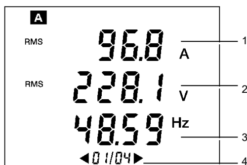
Figure 13 : Exemple d'affichage de la page 1/4.
