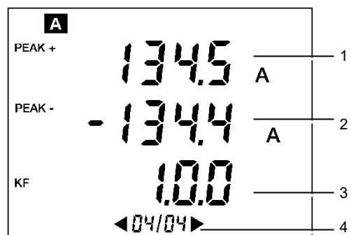
Figure 16 : Exemple d'affichage de la page 4/4.
