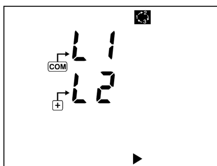
Figure 36 : Le C.A. 8220 est prêt pour la première mesure de détermination de l'ordre des phases.
