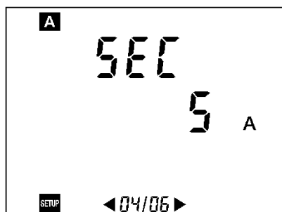
Figure 50 : Affichage du paramètre relatif au courant efficace secondaire du transformateur d'intensité.
