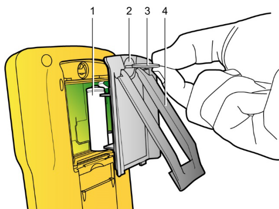
Figure 76 : Accès aux éléments de la batterie.
