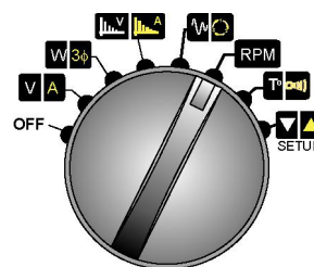
Figure 41 : Le commutateur rotatif en position RPM .
