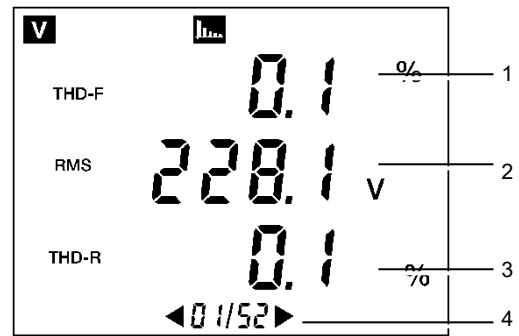
Figure 25 : Exemple d'affichage de la page 1/52.
