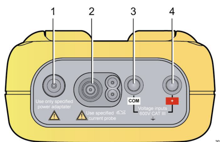
Figure 73 : Les connecteurs en partie supérieure.
