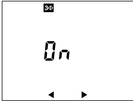
Figure 23 : Dans cet exemple, les calculs concernant le réseau triphasé équilibré sont activés.
