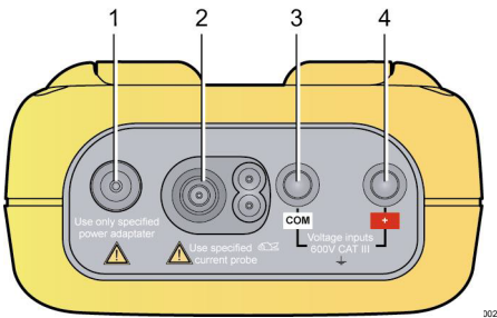
Figure 2 : Les bornes en partie supérieure.
