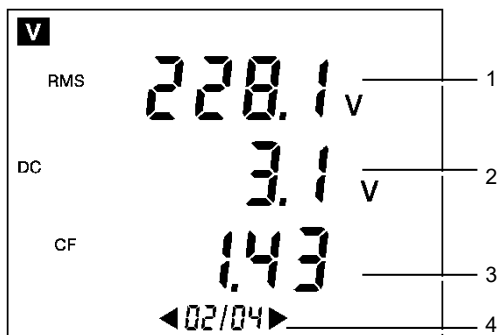
Figure 10 : Exemple d'affichage de la page 2/4.
