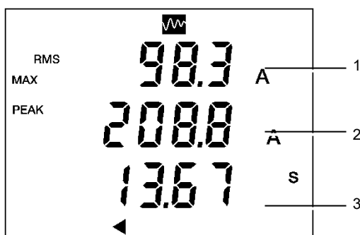
Figure 35 : Exemple d'affichage de résultats.
