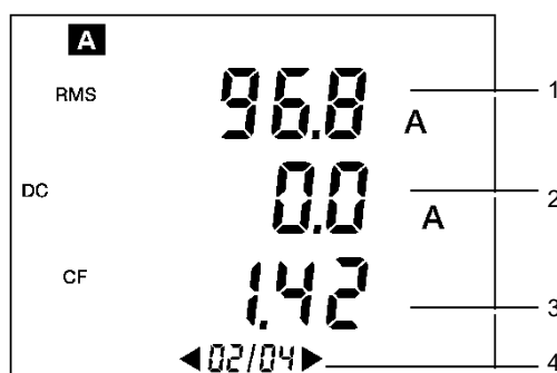
Figure 14 : Exemple d'affichage de la page 2/4.
