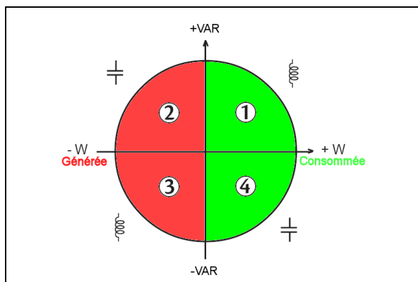
Figure 77 : Représentation des 4 quadrants de puissance.
