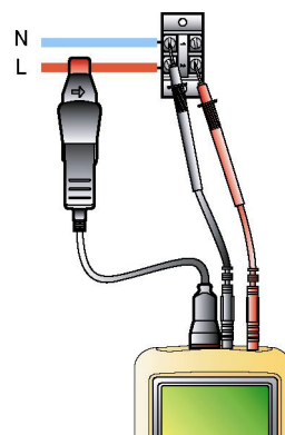
Figure 74 : Connexion en monophasé. 005
