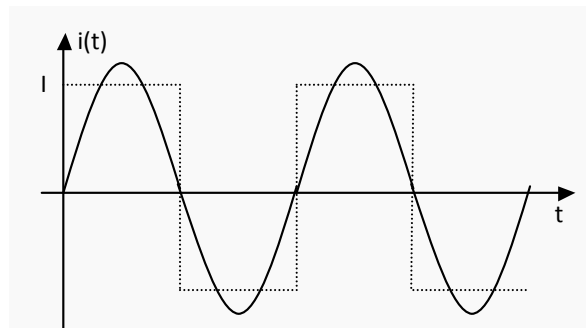
Fig. 9: i(t) rappresentato dal suo fondamentale
